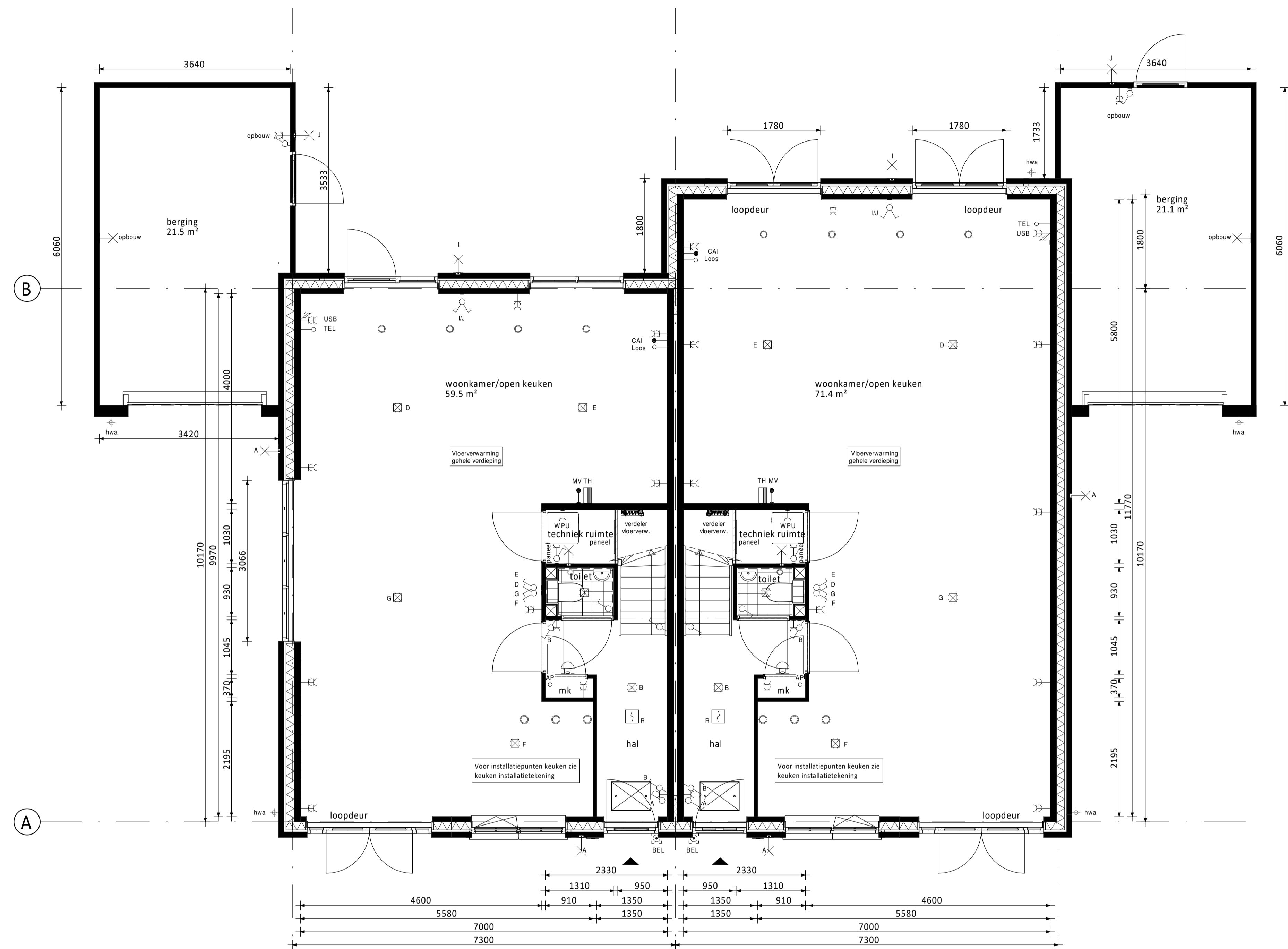
Begane grond
