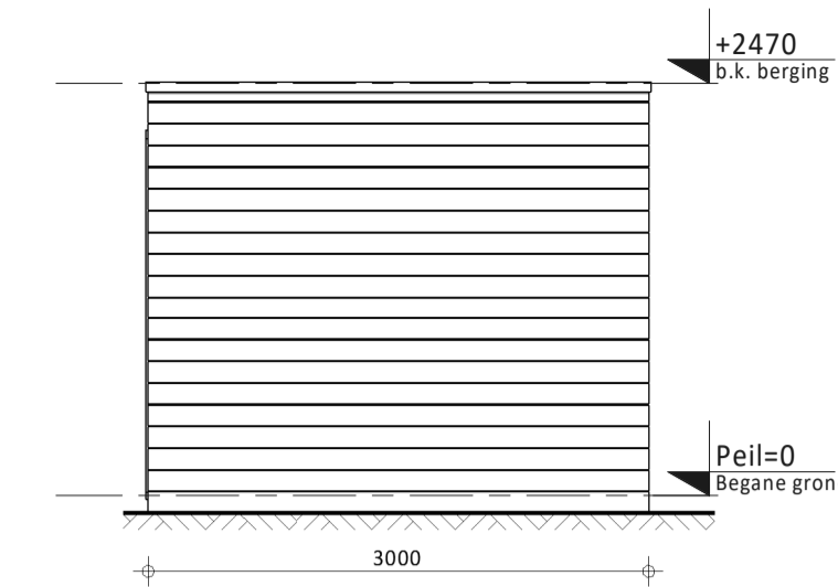
Achteraanzicht
