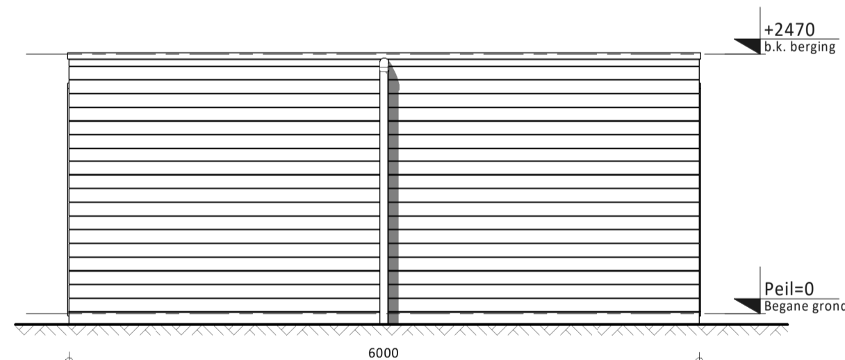
Vooraanzicht
