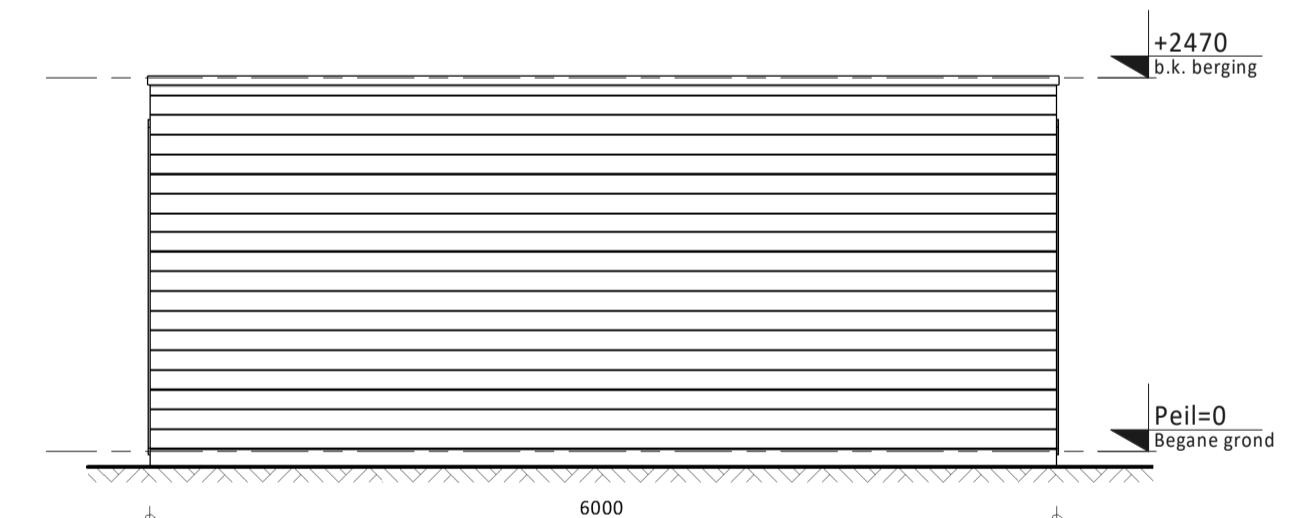
Achteraanzicht
