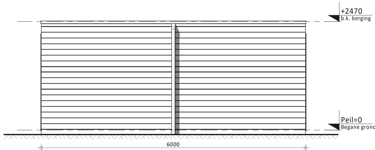
Vooraanzicht
